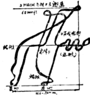
도표 V: 전적인 요격과 초계로서 방공작전을 위한 다용도전투기의 프로파일·및 손(회색 선은 낙하랭크를 장비했을 때)
