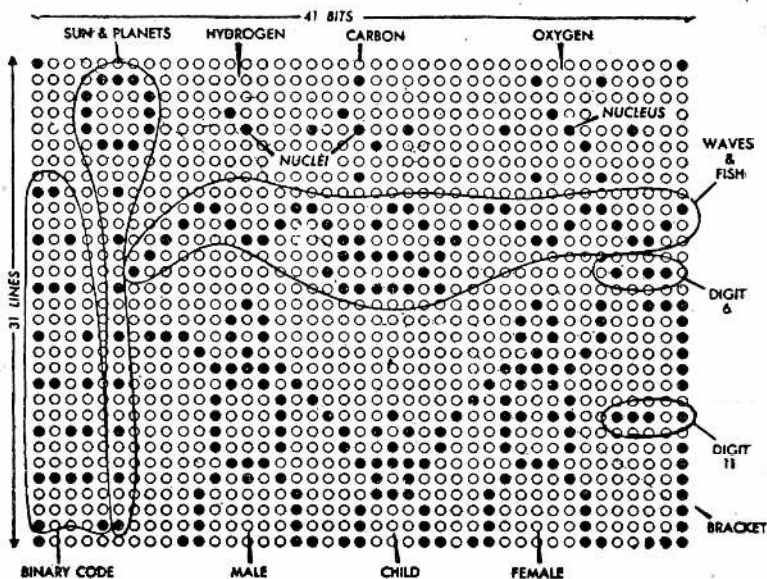
<외계로부터 수신될 신호의 형태>
