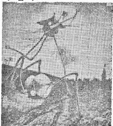
<화성인들의 지구 침공(우주 전쟁에서)>
