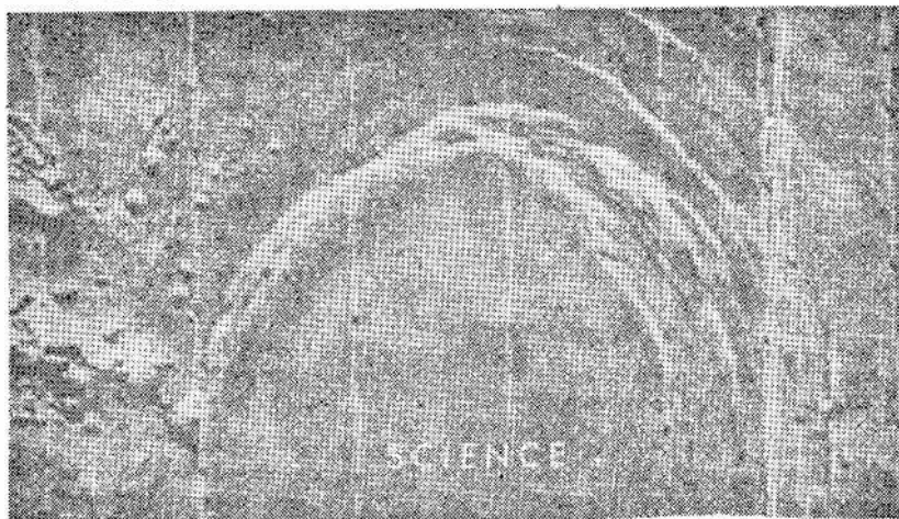
<화성의 적도 근방에 있는 분화구 직경이 약 70마일 가량 된다.>
