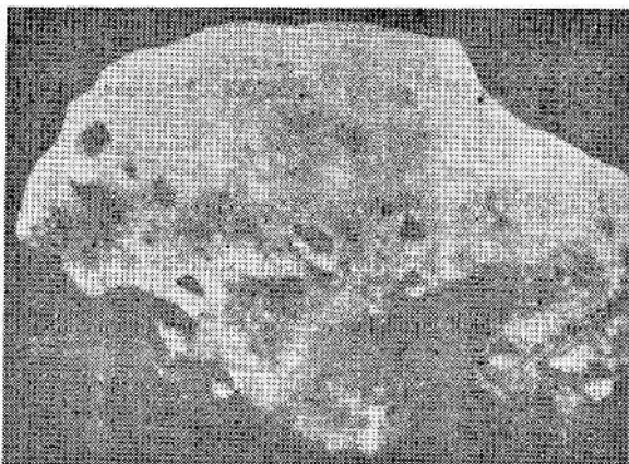
<화성의 달 Phobos의 근접사진. 유성을 얻어 맞아 표면이 곰보같다.>
